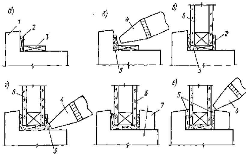
Рис. 8. Установка, крепление и уплотнение стеклопакета в переплете 1 — переплет; 2 — фиксирующая боковая прокладка; 3 — опорная прокладка; 4 — герметизатор; 5 — нетвердеющая мастика; 6 — стеклопакет; 7 — штапик
