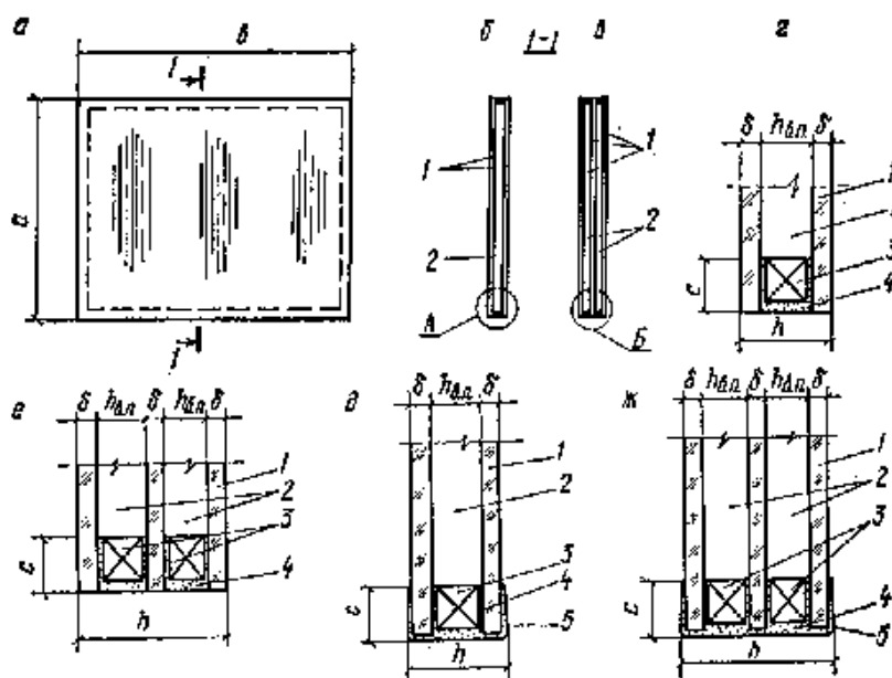
Рис. 4. Конструктивные решения стеклопакетов a — общий вид; б и в — поперечные разрезы двух- и трехслойного стеклопакетов; г и д — схемы соединения стекол в двухслойных стеклопакетах; е и ж — схемы соединения стекол в трехслойных стеклопакетах; 1 — стекло; 2 — воздушная прослойка; 3 — распорная рамка; 4 — клеющая и герметизирующая мастика; 5 — обрамляющая рамка
