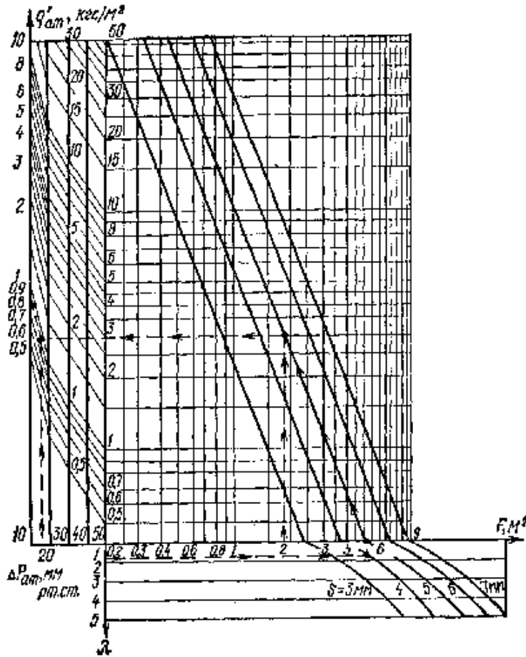
Рис. 2. Номограмма для определения q^I_{ат}
